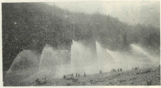
角野橋下流での放水試験
